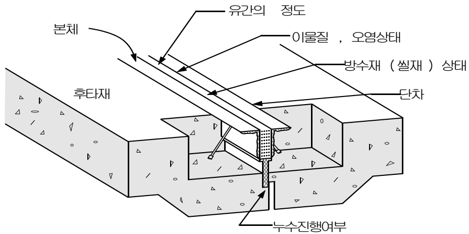
< 신축이음 점검부위 >
